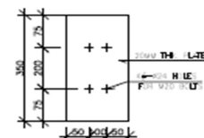
DET-ILS FOR SP-4
