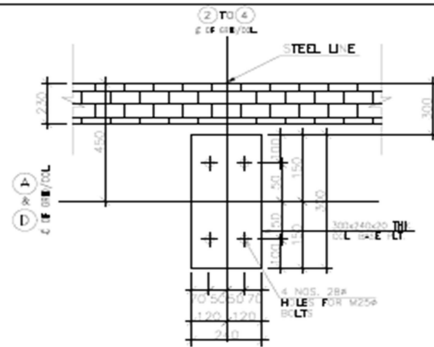
DETAIL B (06 Nos. REOD.)
